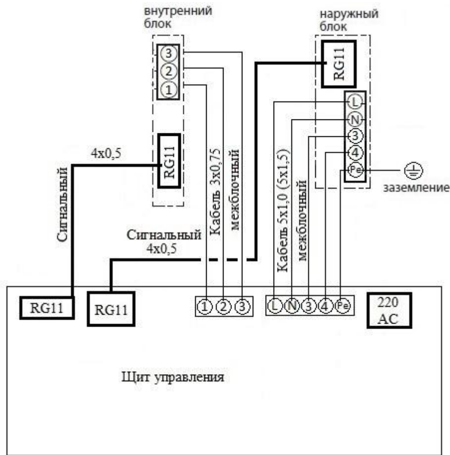
Рис 2. Электрическая схема подключения холодильной машины
